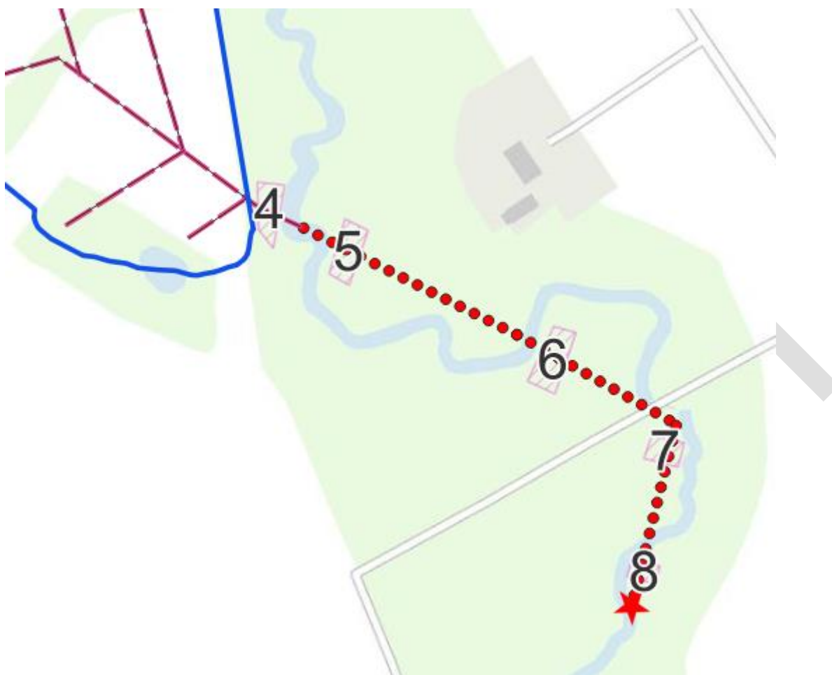
Kort 4.6.1: Kort over det dræn der afvander hel projektområdet via dræn til Krobæk (rød stiplede linje). Rørledningens placering er ikke kendt, men rørets udløb kendes (markeret med stjerne).
