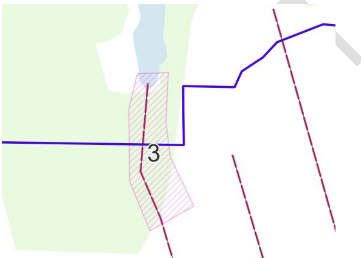
Kort 4.5.1: Kort over undersøgelses- og arbejdsområde 3. Afløb fra søen sker via overløb til dræn med styrtfald. (drænen er markeret med rød stiplede linje, projektgrænse med blå og undersøgelsesområde skraveret)
