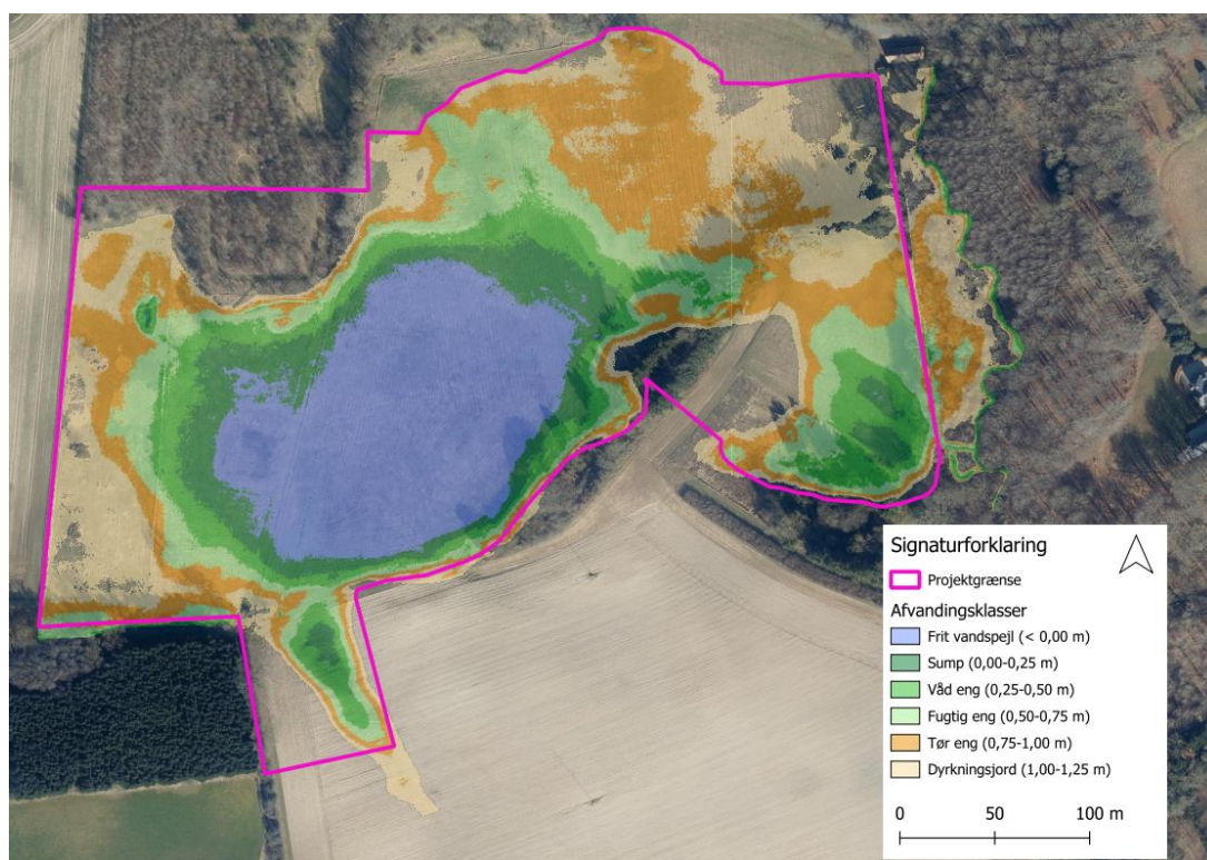
Kort 7.3: Afvandingskort projekteret sommerkiddel.
