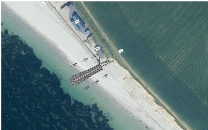
Plantegning af høfden, der viser placeringen samt tværsnit af høfden. Tallene angiver afstanden til henholdsvis bebyggelsen på Strandvej 31
